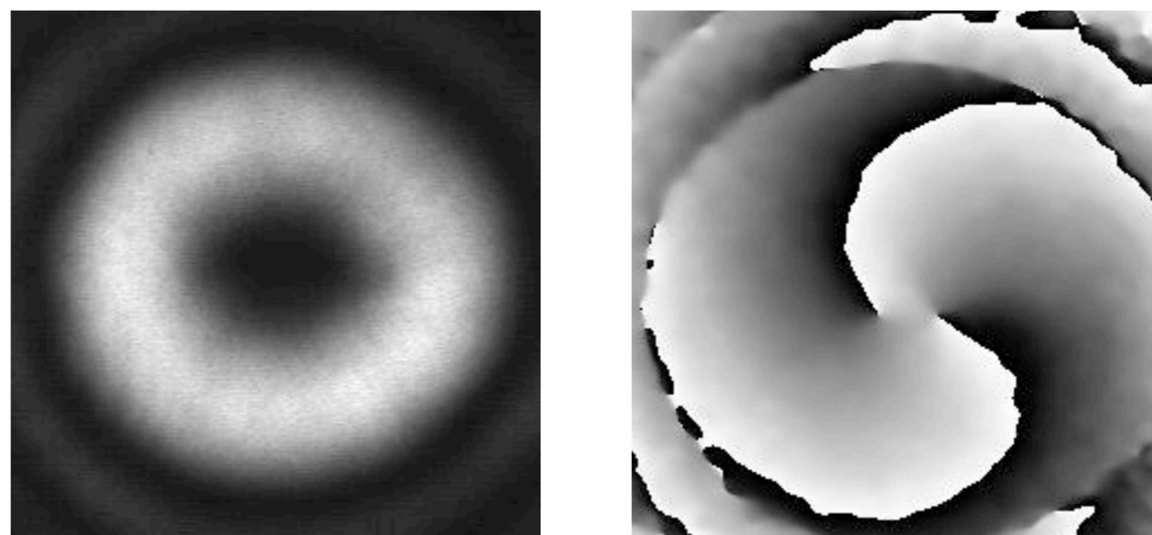
ラゲールガウスビーム (m=2) の強度分布 (左) と位相分布
